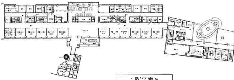
4階平面図
